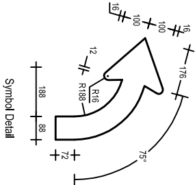
W1-3A(L) 600 x 600
